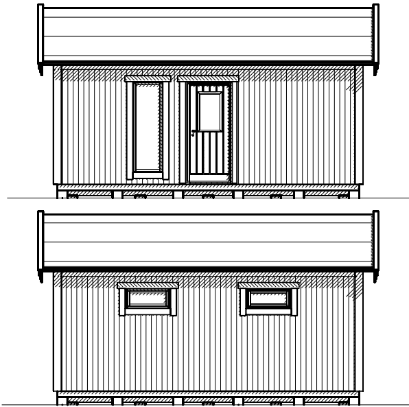
Långsida
